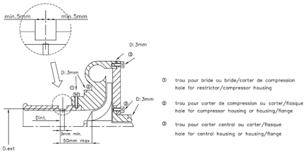
TEKENING 253-65
